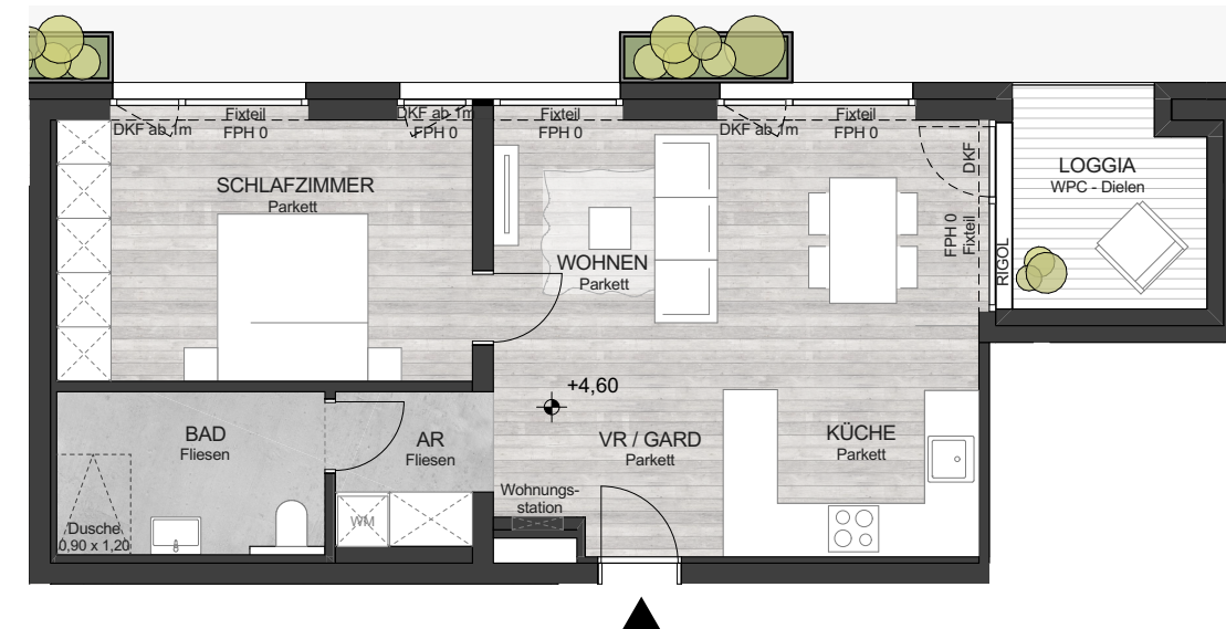
2. OG
