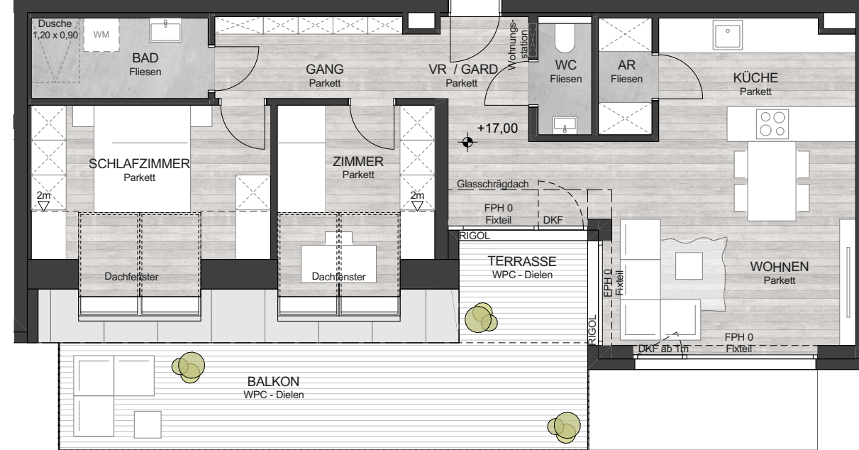
1. DG
