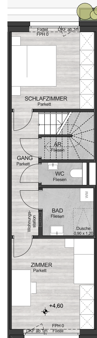
2. OG
