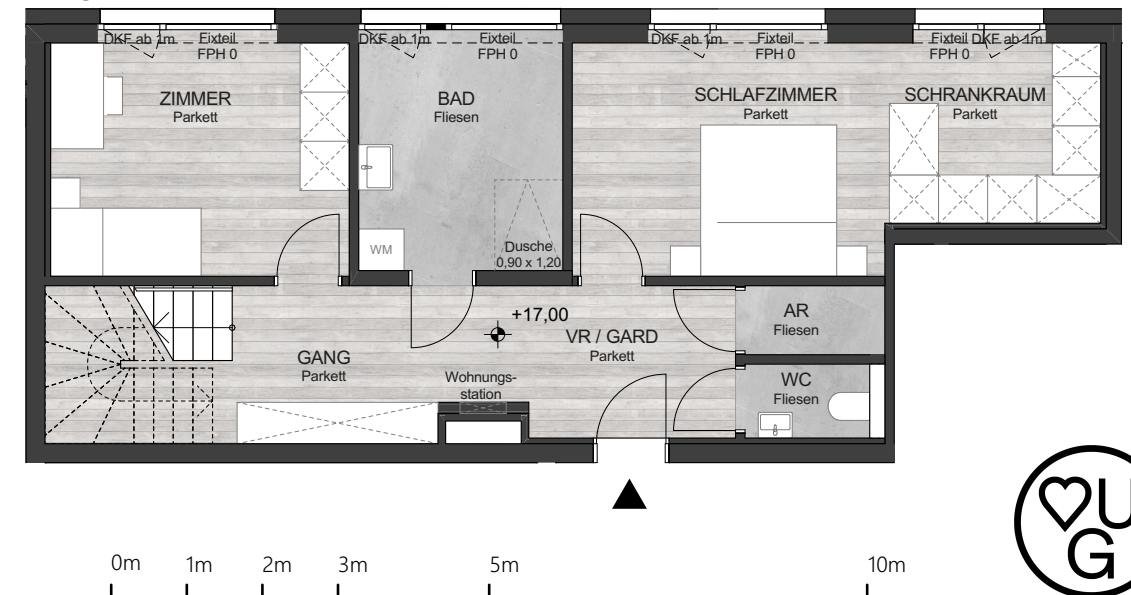
1.DG
