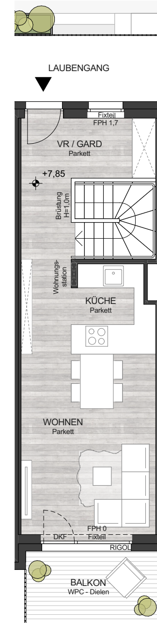
3. OG
